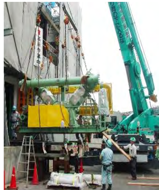
酸素ガス圧縮機据付
